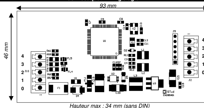
Hauteur max : 34 mm (sans DIN)
